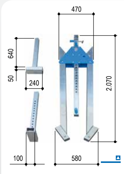
Katlı yan şasi
